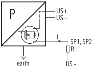
Conexión de cargas a la salida de conmutación
